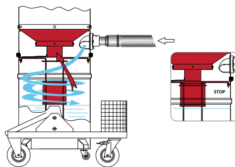
Optional - Arresto meccanico per liquidi
